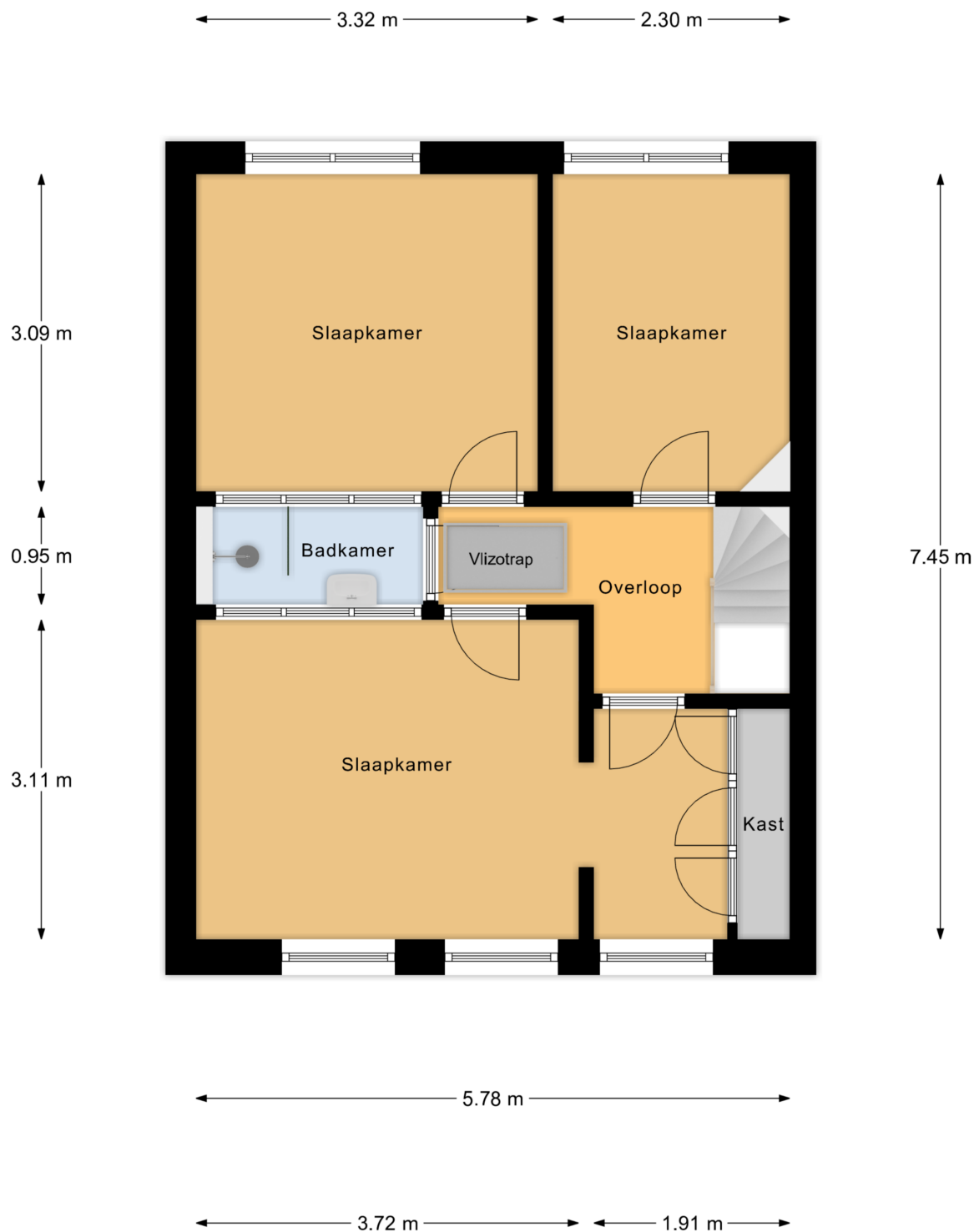
1e Verdieping
