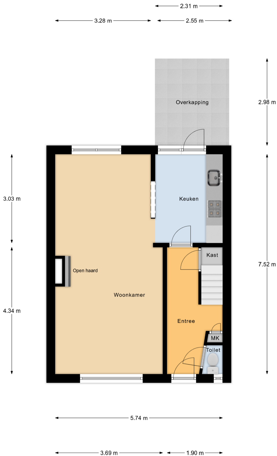
Begane Grond
