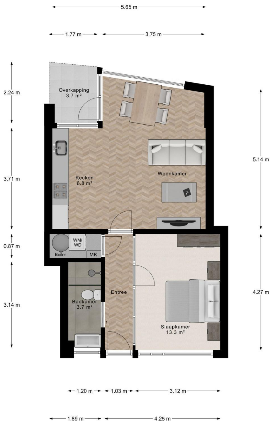
Begane Grond
