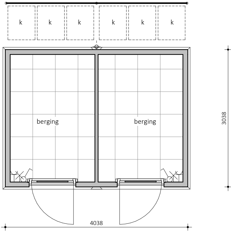
Begane grond
