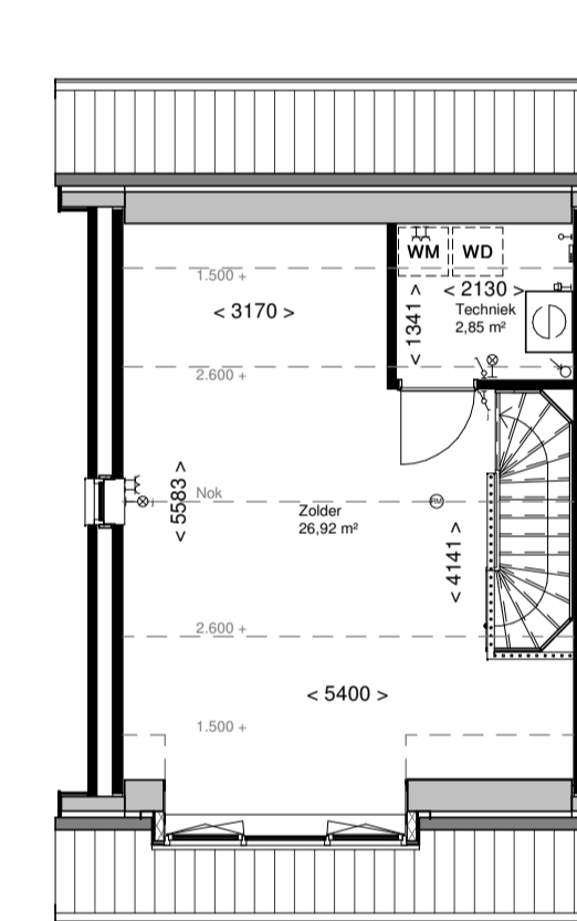
R 512 Dakkapel breedte ca. 3200mm
