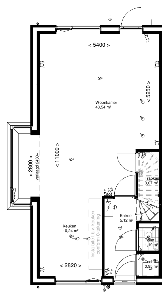
R 202 Achteruitbouw van 2400mm
