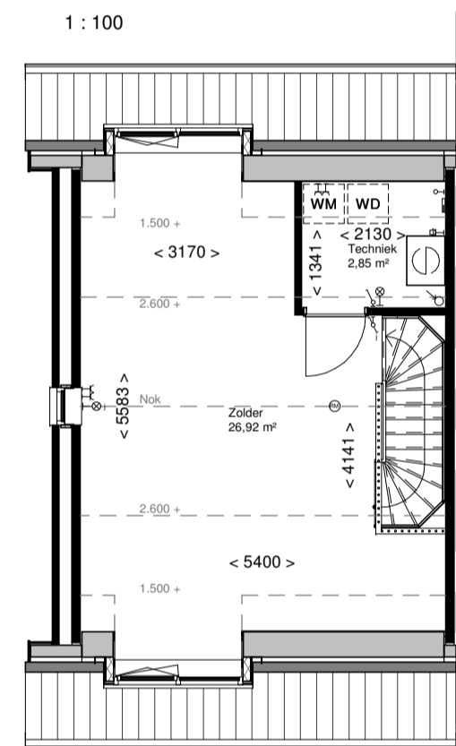
R 511 Dakkapel breedte ca. 2200mm
