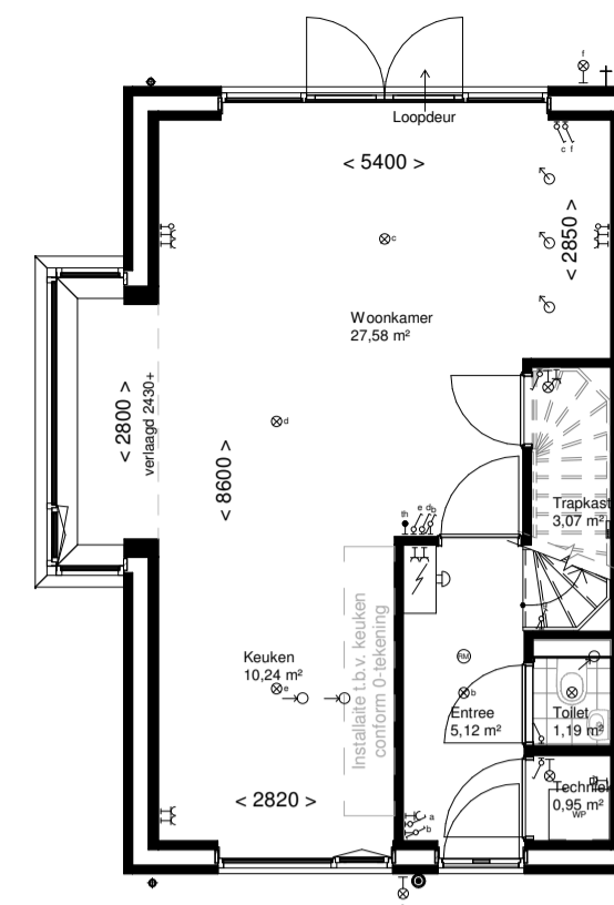
R 302 Dubbele tuindeuren met zijlichten i.p.v. vast glas
