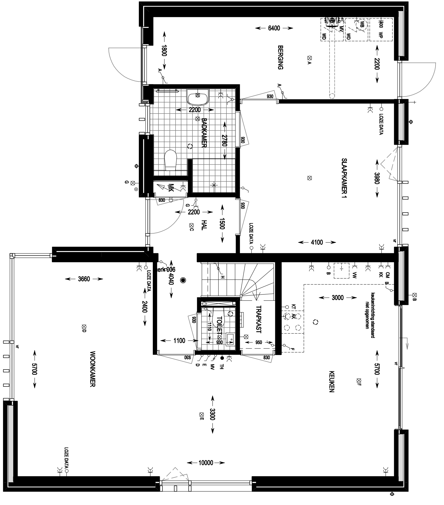
begane grond bouwnummer 43
